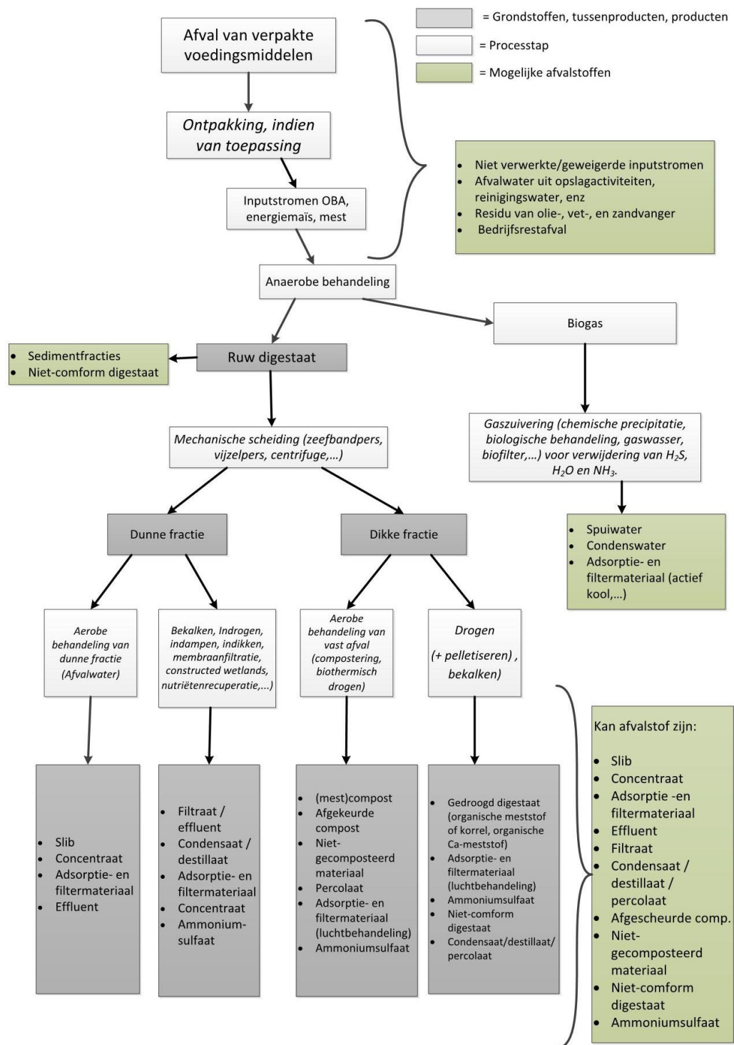
Figuur 1. Schematisch overzicht van het vergistingsproces met focus op de afvalstromen.
